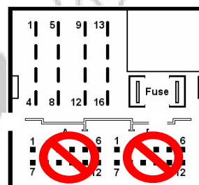
MOST Anschluss am Navi
